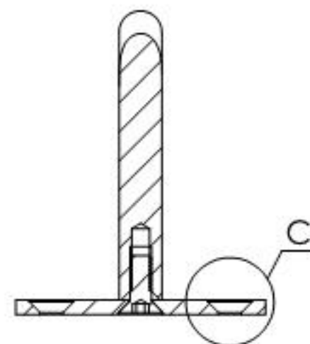
SCHNITT B-B
