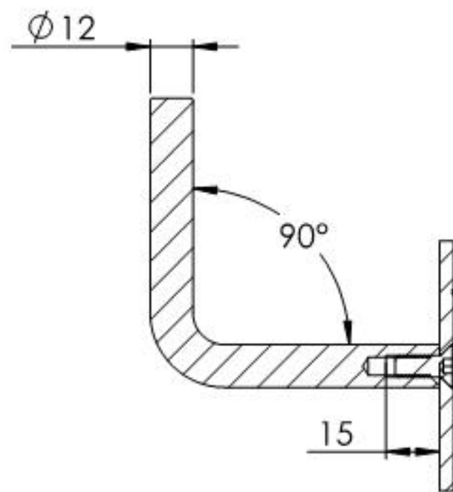
SCHNITT A-A
