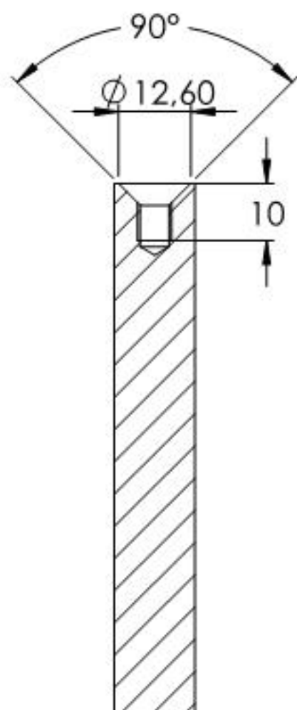
SCHNITT C-C
