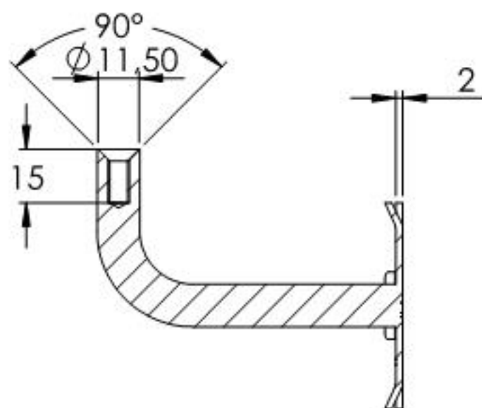
SCHNITT A-A
