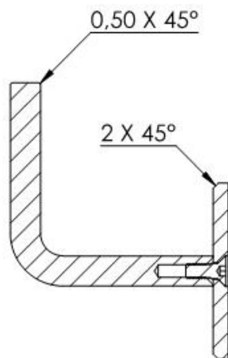
SCHNITT A-A
