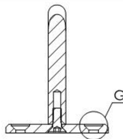
SCHNITT B-B
