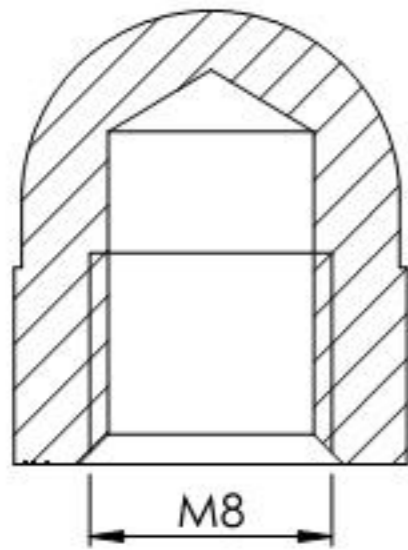
SCHNITT A-A
