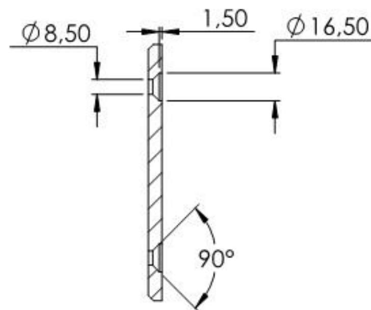
SCHNITT A-A
