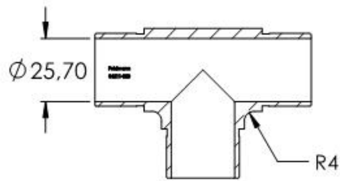
SCHNITT A-A
