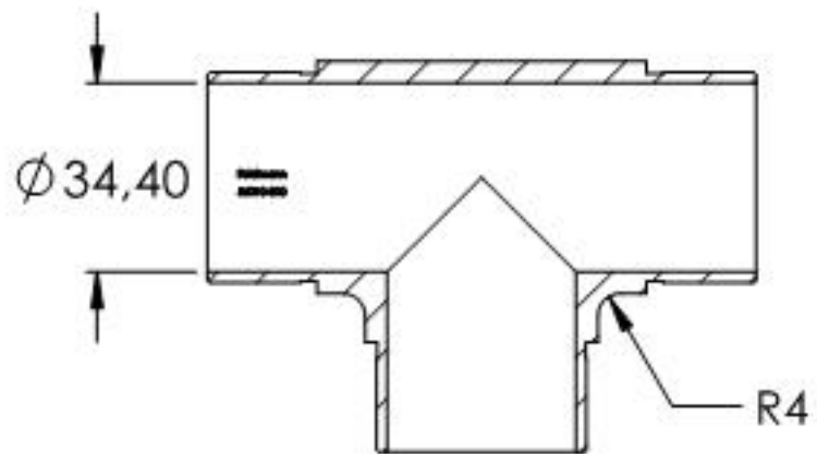
SCHNITT A-A
