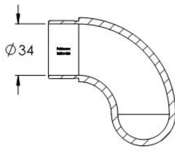
SCHNITT A-A
