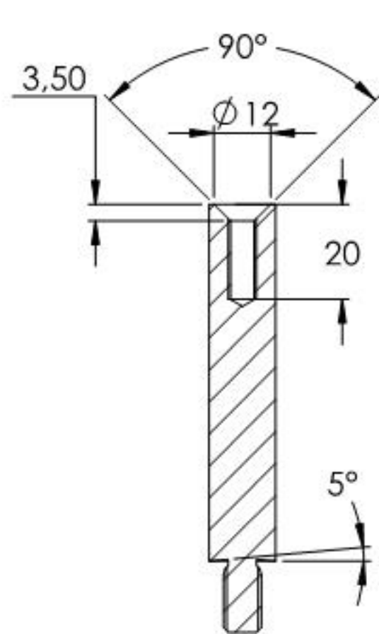
SCHNITT A-A
