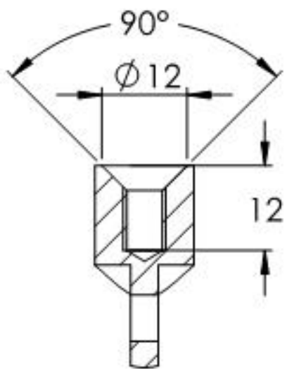
SCHNITT B-B
