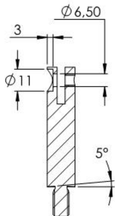
SCHNITT A-A
