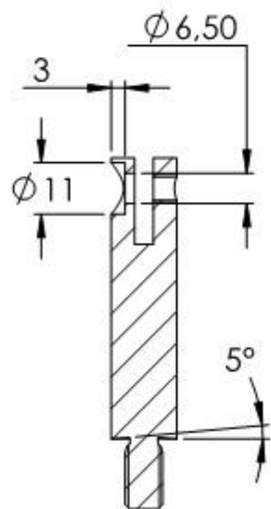
SCHNITT A-A
