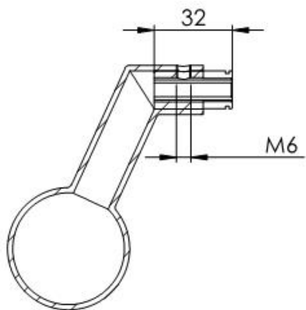
SCHNITT A-A
