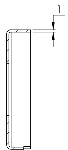
SCHNITT B-B
