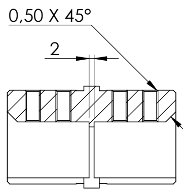
SCHNITT A-A
