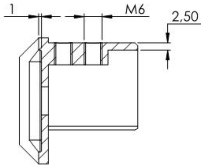
SCHNITT A-A
