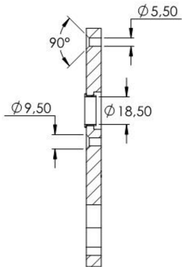
SCHNITT A-A
