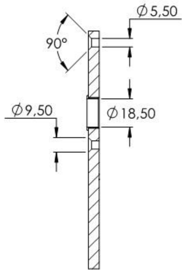
SCHNITT A-A
