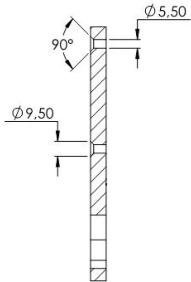
SCHNITT A-A
