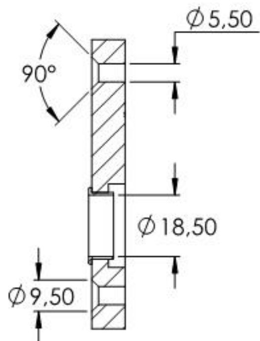
SCHNITT A-A
