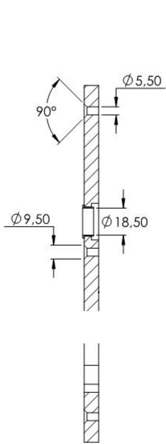
SCHNITT A-A
