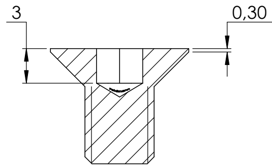
SCHNITT A-A
