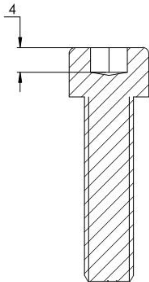
SCHNITT A-A
