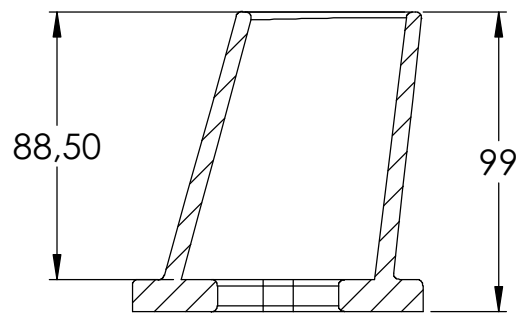
SCHNITT A-A
