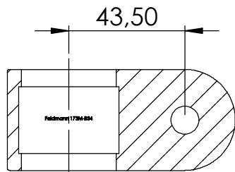
SCHNITT A-A
