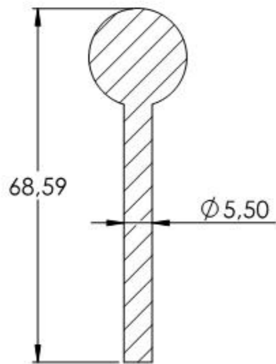
SCHNITT A-A
