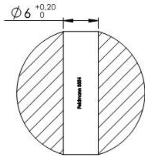
SCHNITT A-A
