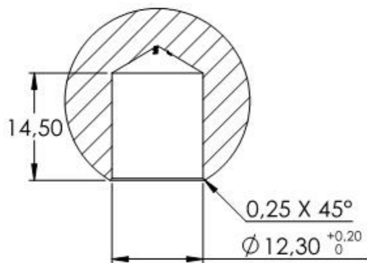
SCHNITT A-A
