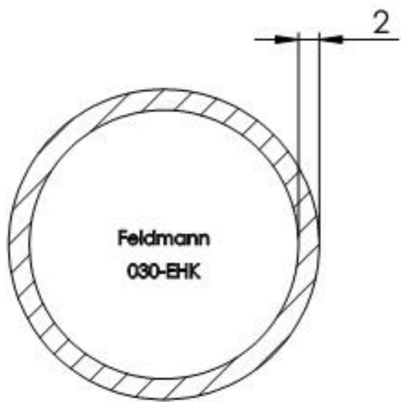
SCHNITT A-A
