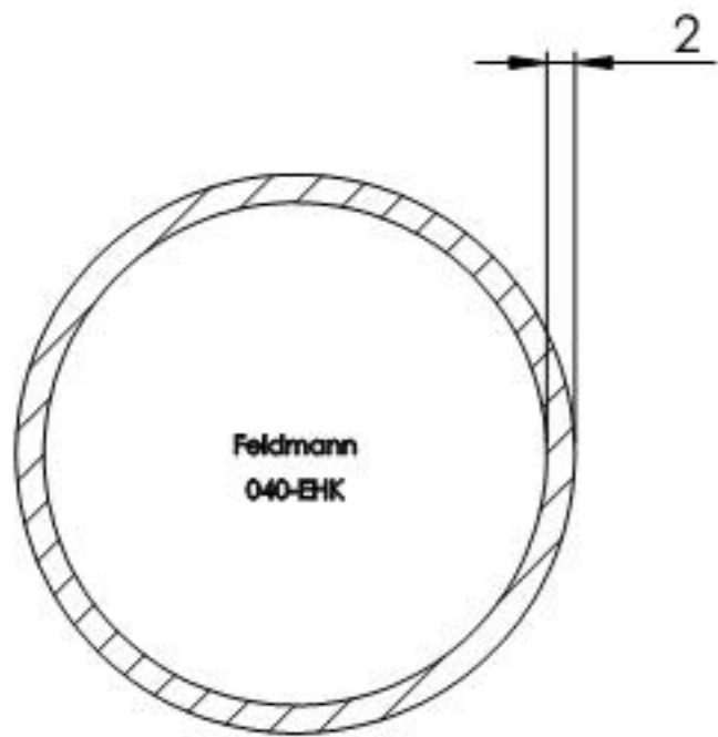
SCHNITT A-A
