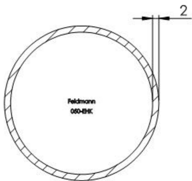
SCHNITT A-A
