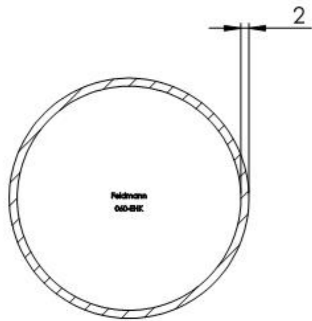
SCHNITT A-A
