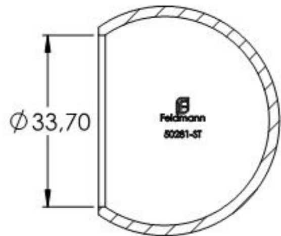
SCHNITT A-A
