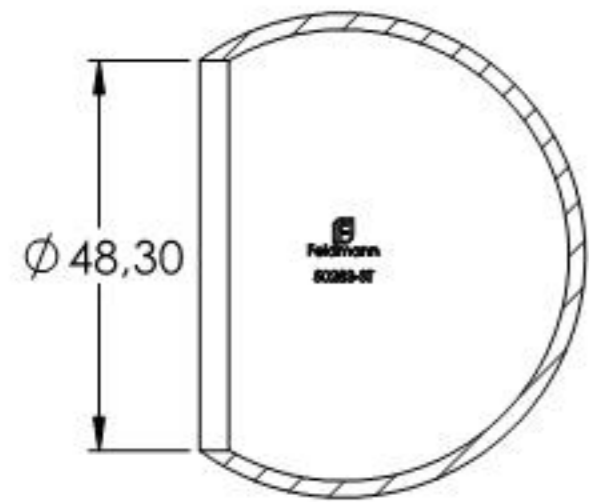
SCHNITT A-A
