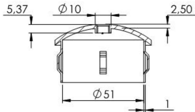
SCHNITT A-A
