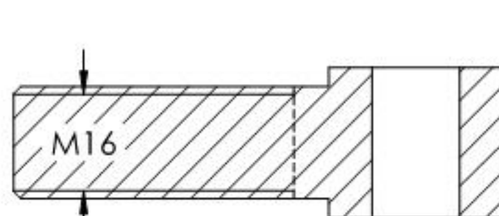
SCHNITT B-B
