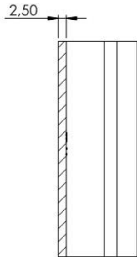
SCHNITT B-B
