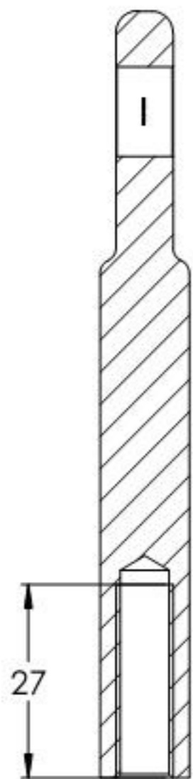
SCHNITT A-A
