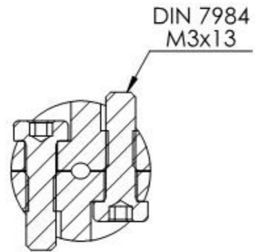
SCHNITT A-A
