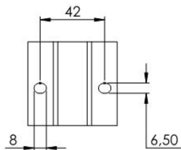
B (1 : 2)
