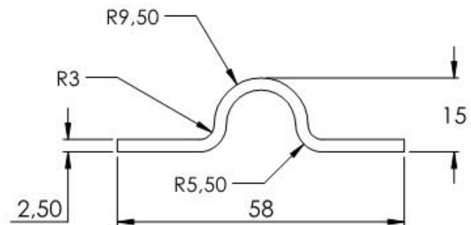
A (1 : 1)
