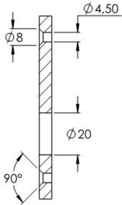
SCHNITT A-A
