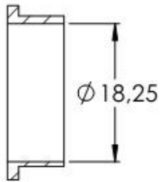
SCHNITT B-B
