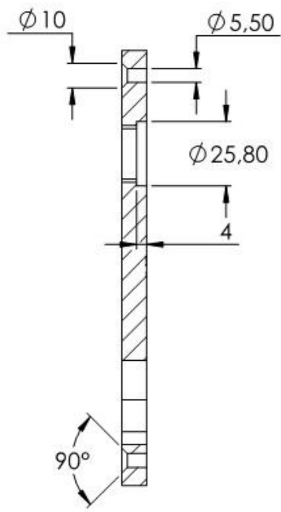
SCHNITT A-A
