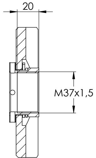
SCHNITT A-A
