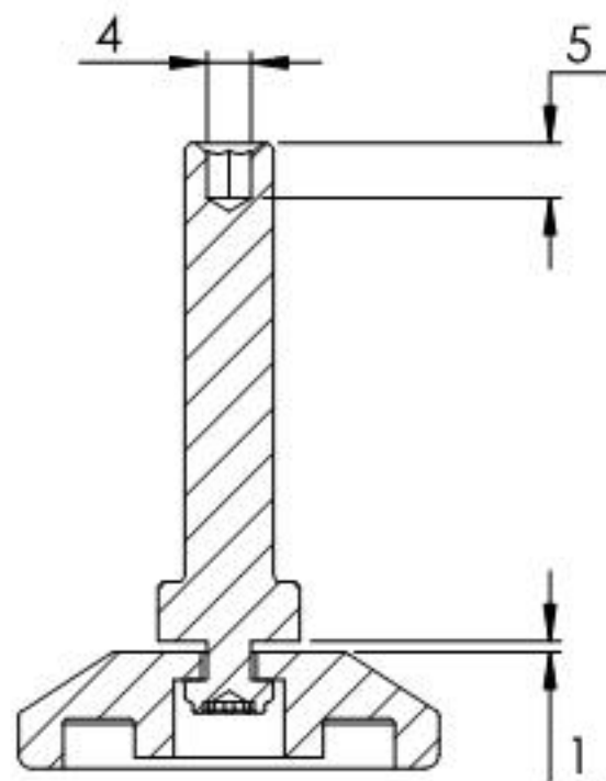
SCHNITT A-A
