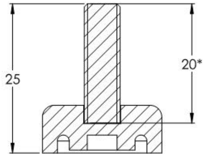
SCHNITT A-A
