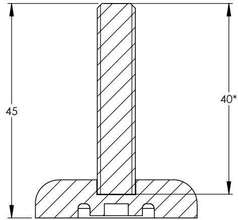
SCHNITT A-A
