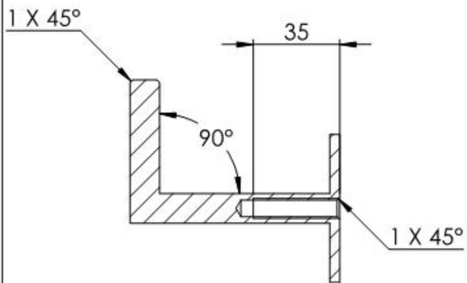
SCHNITT A-A
