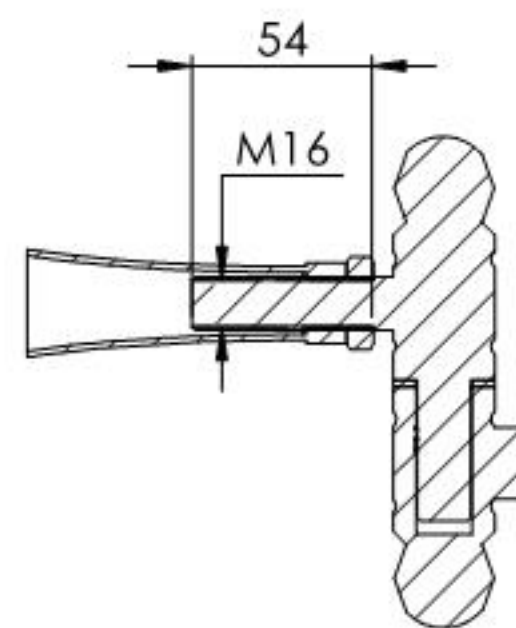
SCHNITT A-A
