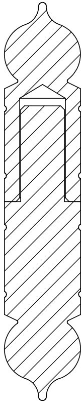
SCHNITT A-A
