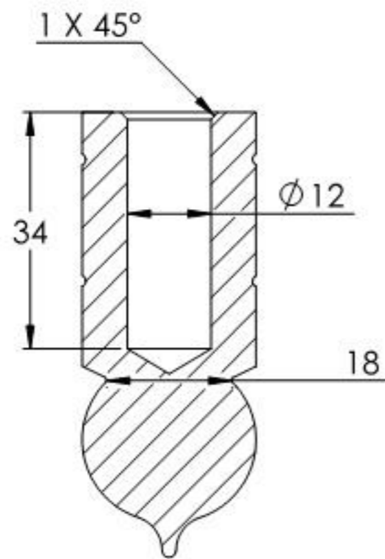
SCHNITT C-C
